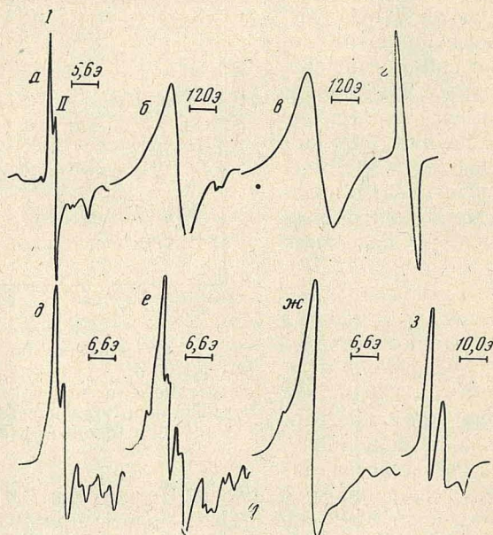
Рис. 4. Спектры ЭПР K_2S_2O_8 при T = 77^\circ K : а — послевзрывной образец, I - g \approx 2,0041 , II - g \approx 2,0039 , \Delta H = 14 э; б — послевзрывной образец, прогретый при T \approx 200^\circ C ; в — образец из верхней части контейнера при V_i / V_0 = 0,4 ; г — послевзрывной образец, облученный рентгеновыми лучами; д — образец, облученный \gamma -лучами, g \approx 2,004 , \Delta H = 9,7 э; е — образец, облученный рентгеновыми лучами, g \approx 2,004 , \Delta H = 9,8 э; ж — образец, облученный и прогретый при T \approx 200^\circ C ; з — образец, облученный \gamma -лучами и ударно-сжатый, g \approx 2,0088 , \Delta H = 9,5 э
